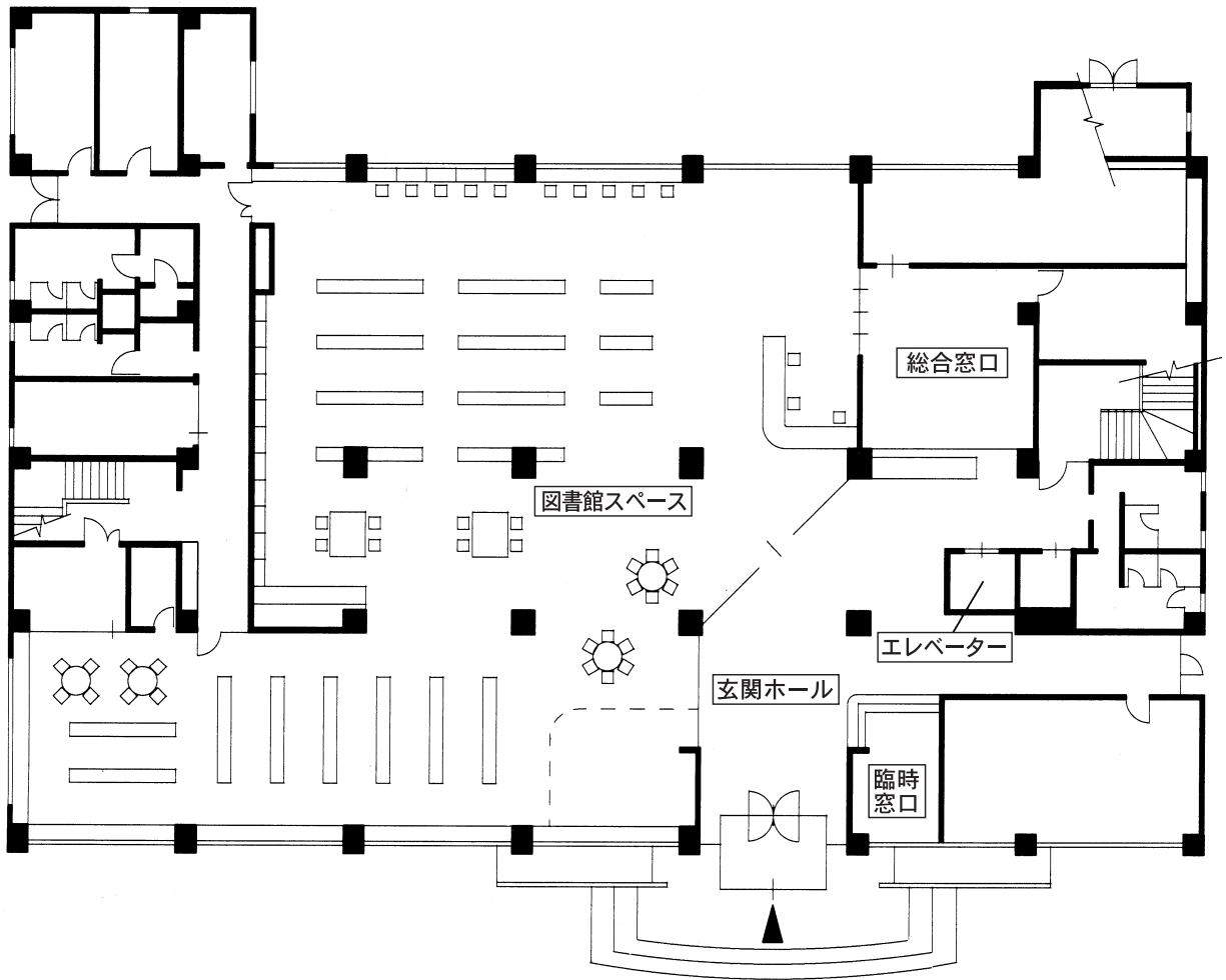
一階 図書館平面図
